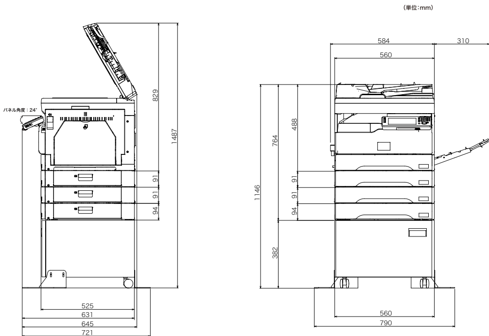
標準 + 給紙ユニット(L)×3段 + 専用台Lowタイプ + 固定脚
