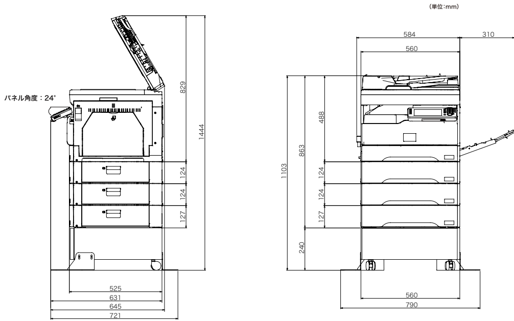
標準 + 給紙ユニット(L)×3段 + 専用台Lowタイプ + 固定脚
