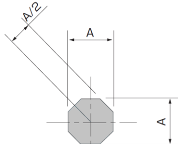
正八角形
