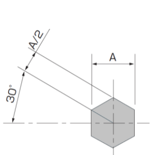
正六角形
