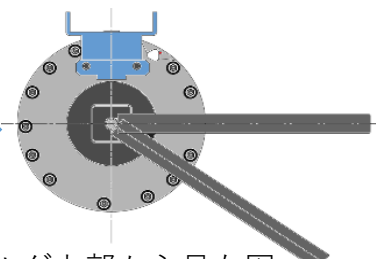
パンチホルダ上部から見た図
